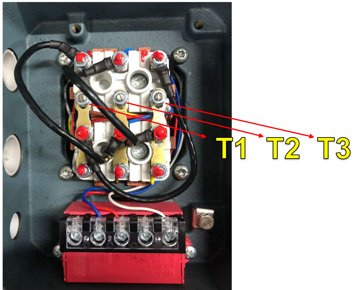
Exemplo de ligação 220v
